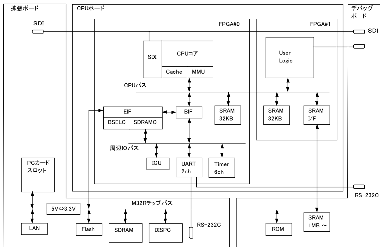
図 8 評価用ターゲットボード (Mappi) の構成
