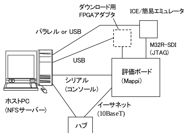
図 9 ソフトウェア開発・デバッグ環境
