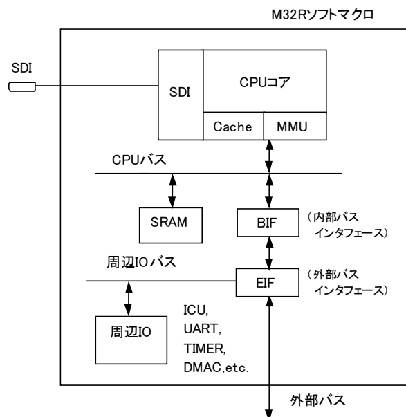
図4 M32R ソフトマクロの構成
