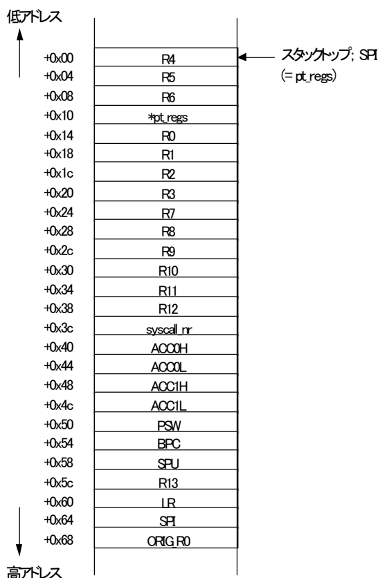
図 6 システムコール発行時のスタック・フレーム
