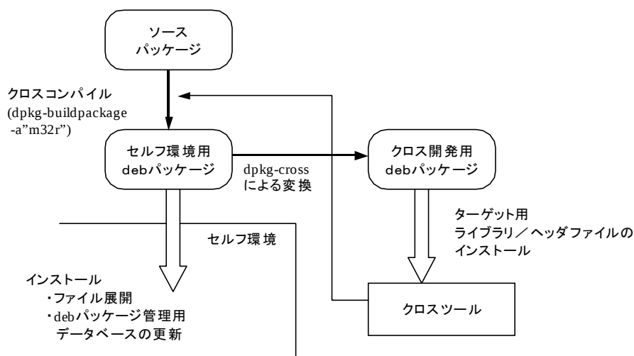
図 10 deb パッケージを利用したクロス開発の流れ
