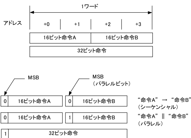
図3 命令フォーマット
