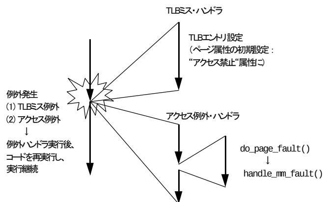
図 7 例外発生とデマンドローディング処理
